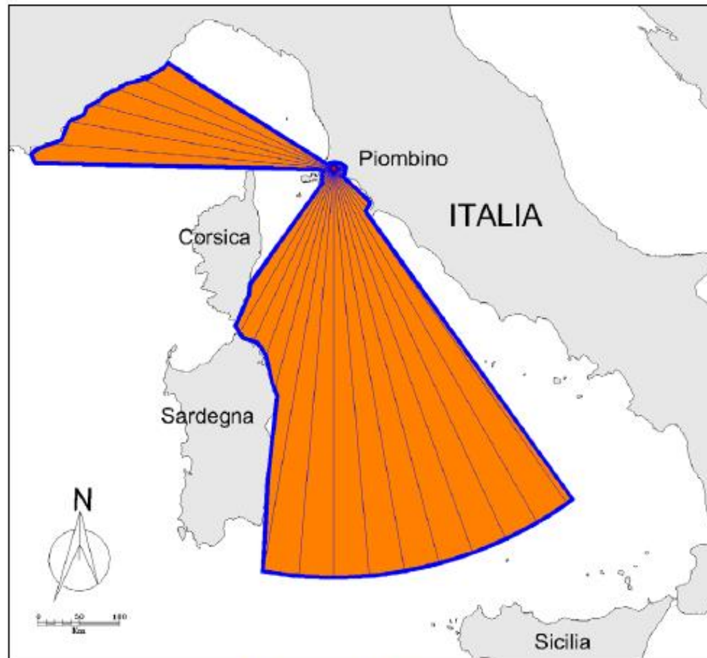
Figura 2.2: Fetch geografici al largo di Piombino.
