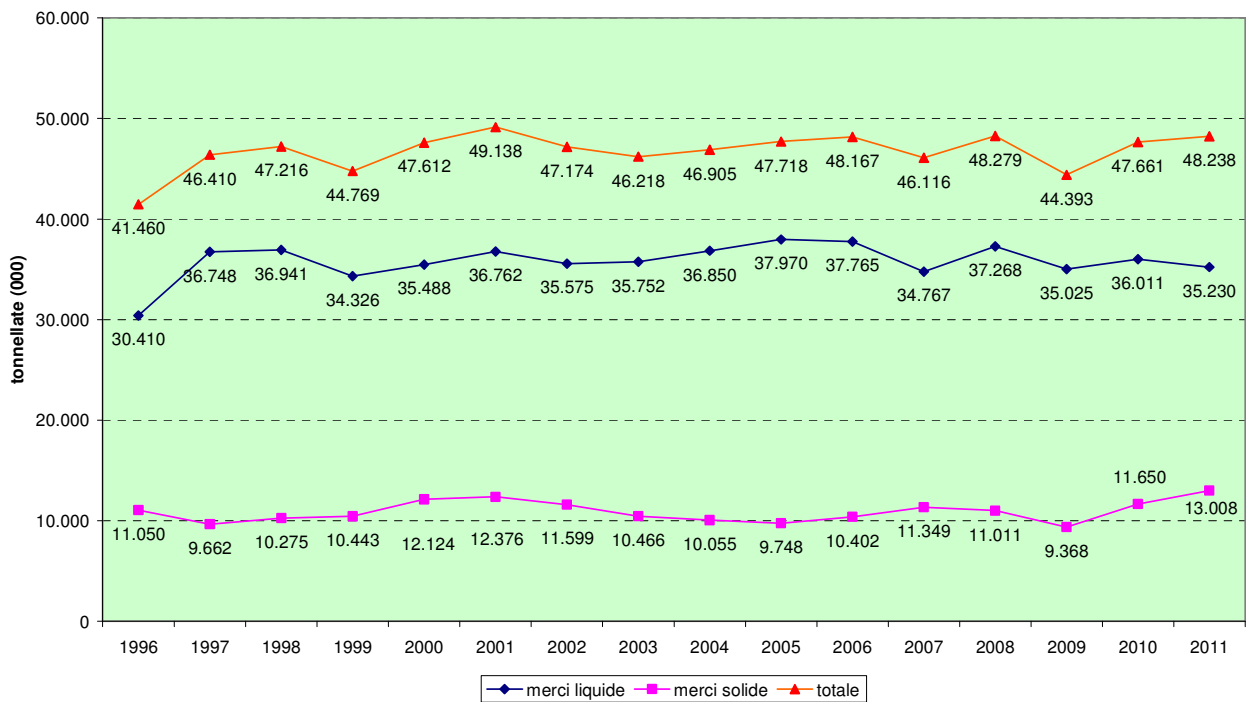
AP Trieste - Merci movimentate distinte in liquide e solide - Anni 1996-2011
