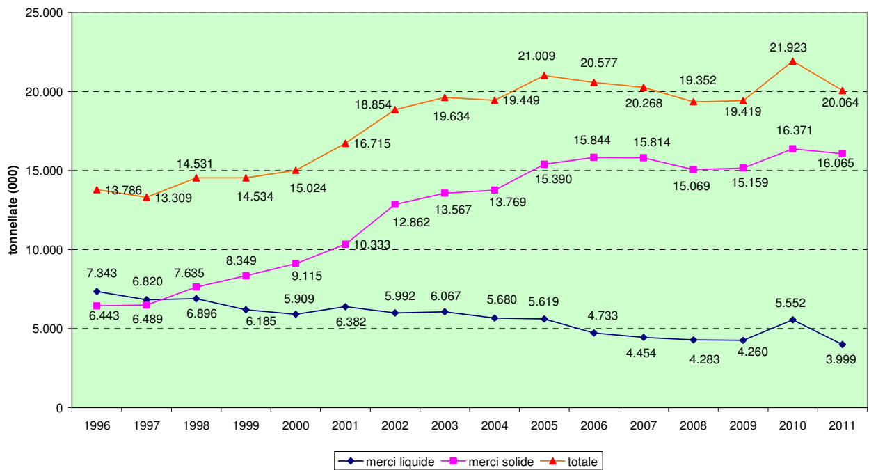
AP Napoli - Merci movimentate distinte in liquide e solide - Anni 1996-2011
