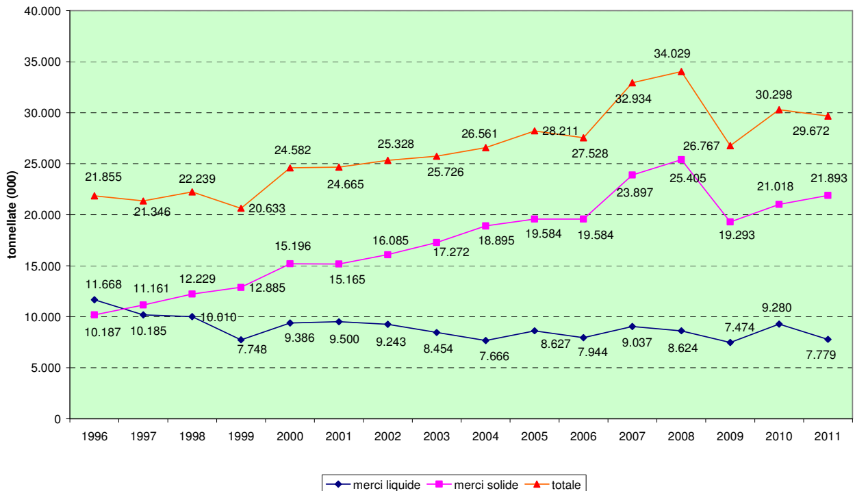
AP Livorno - Merci movimentate distinte in liquide e solide - Anni 1996-2011
