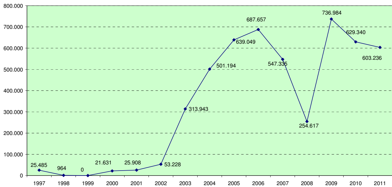
AP Cagliari-P. Foxi - Contenitori movimentati - Anni 1996-2011
