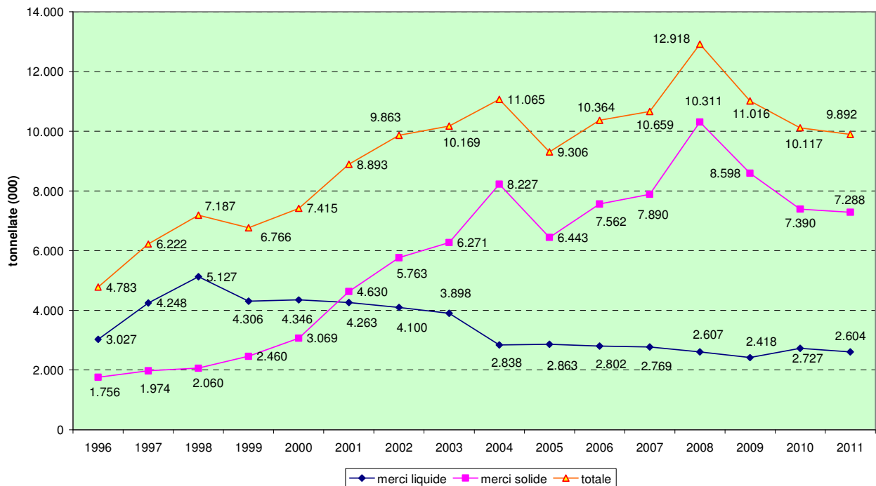
AP Brindisi - Merci movimentate distinte in liquide e solide - Anni 1996-2011
