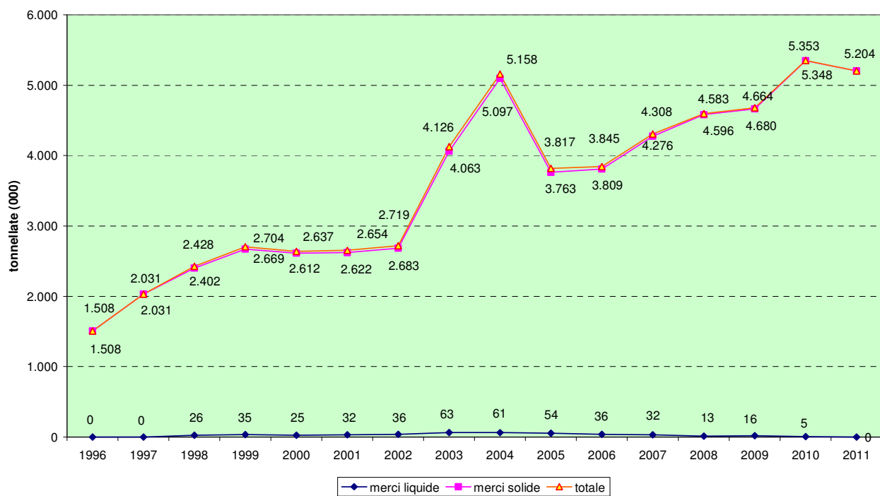
AP Catania - Merci movimentate distinte in liquide e solide - Anni 1996-2011
