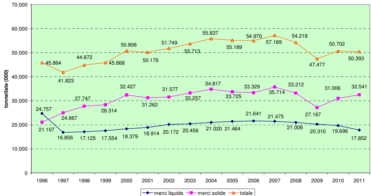
AP Genova - Merci movimentate distinte in liquide e solide - Anni 1996-2011
