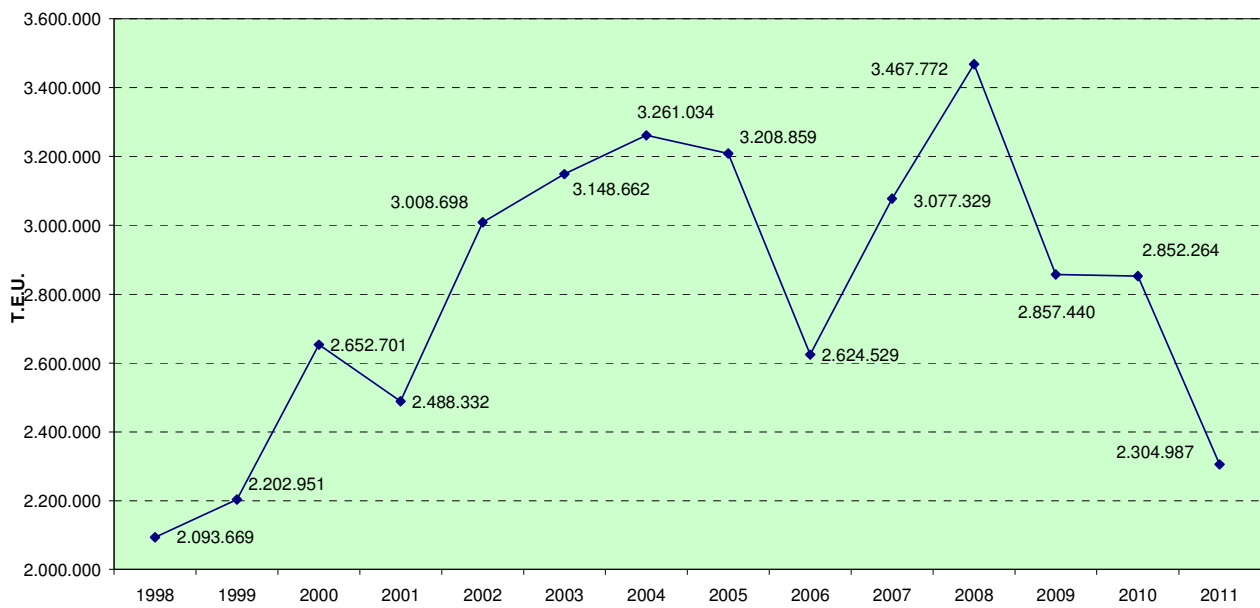
AP Gioia Tauro - Contenitori movimentati - Anni 1998-2011
