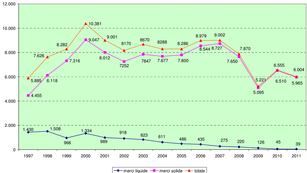
AP Piombino-Portoferraio - Merci movimentate distinte in liquide e solide - Anni 1997-2011
